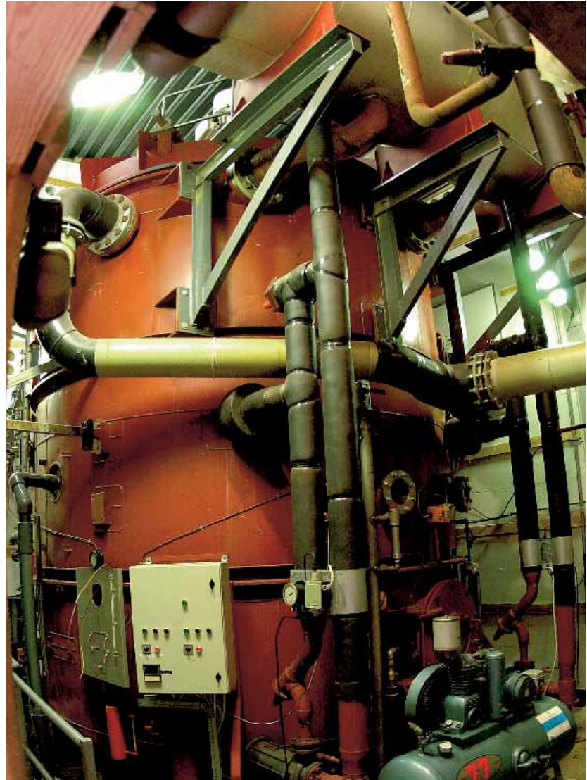
Vakuamtanken, hvor vakuum opretholdes tæt ved vandets triplepunkt, så en del af vandet omgænder til is. Herved frigives frysevarmen, der omdanner tilsvarende mængde vand til damp. Fordampningsvarmen genindvindes og udnyttes til fjernvarmevand.
